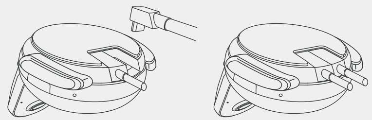
Cable OBD QuickConnect con la iQ
